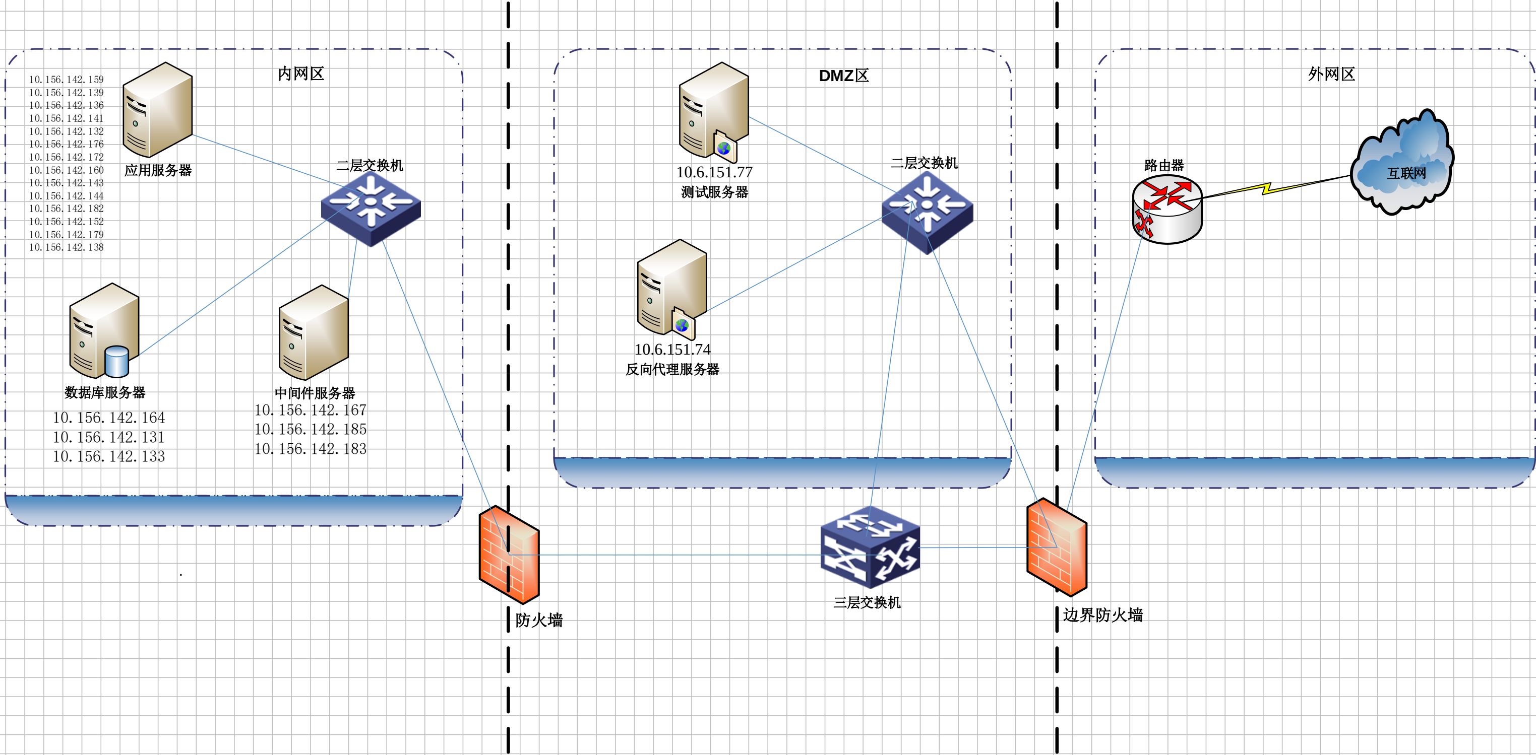
人员定位系统部署拓扑图
